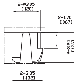
DET.A SCALE 2:1
